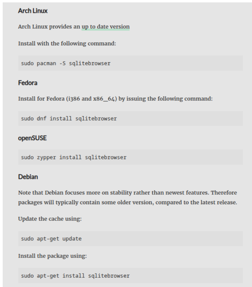
Figure 3: Komendy instalacyjne dla najpopularniejszych dystrybucji
