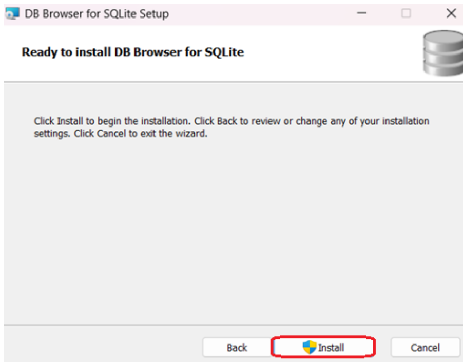
Figure 7: Instalacja
