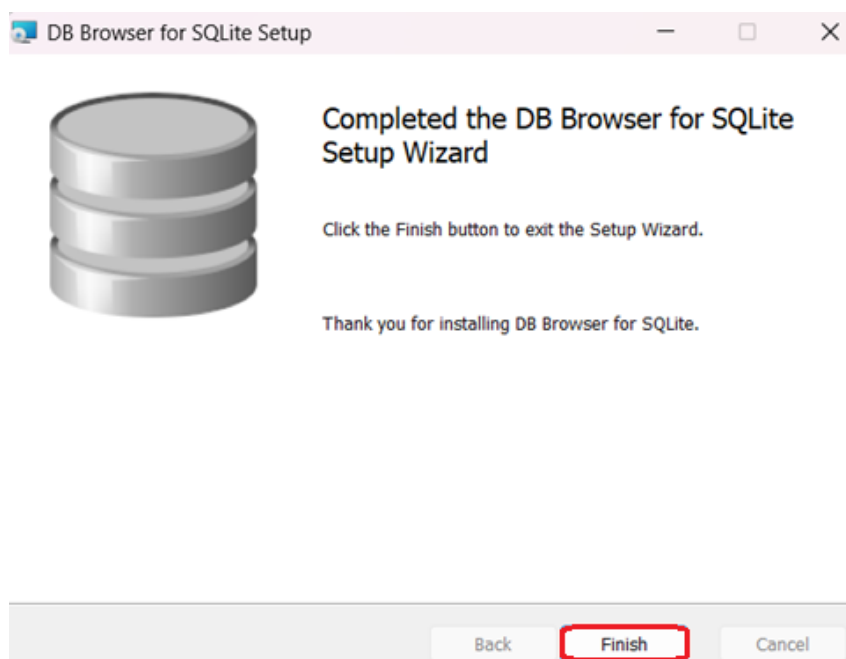
Figure 9: Koniec instalacji
